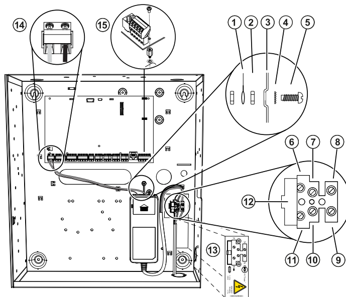
Abbildung 10: HS3032/HS3128/HS3248 in Verdrahtung HSC3010C (Argentinien)
