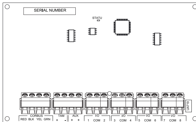
Abbildung 23: HSM3408 8-Linienerweiterung
