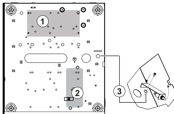
Abbildung 5: HSM3204CX/HSM3350 in Gehäusen von HSC3010C, HSC3010CR, HSC3030CAR montiert
