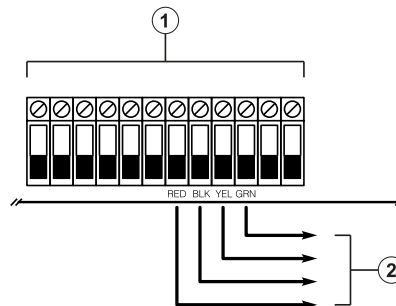
Abbildung 26: HSM2HOSTx Verkabelungsdiagramm
