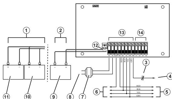
Abbildung 27: HSM2300/2204 Verkabelung der Stromversorgung
