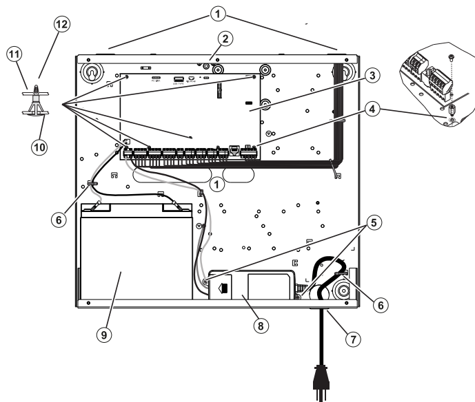
Abbildung 11: Verkabelung der Zentrale für HSC3020C (für Nordamerika)
