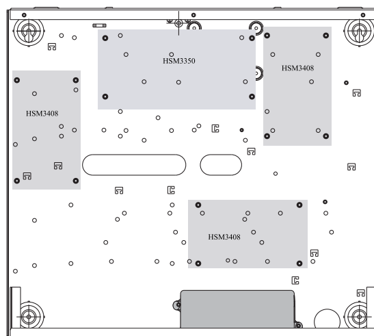
Abbildung 7: Module HSM3408 und HSM3350 im Gehäuse HSC3020C
