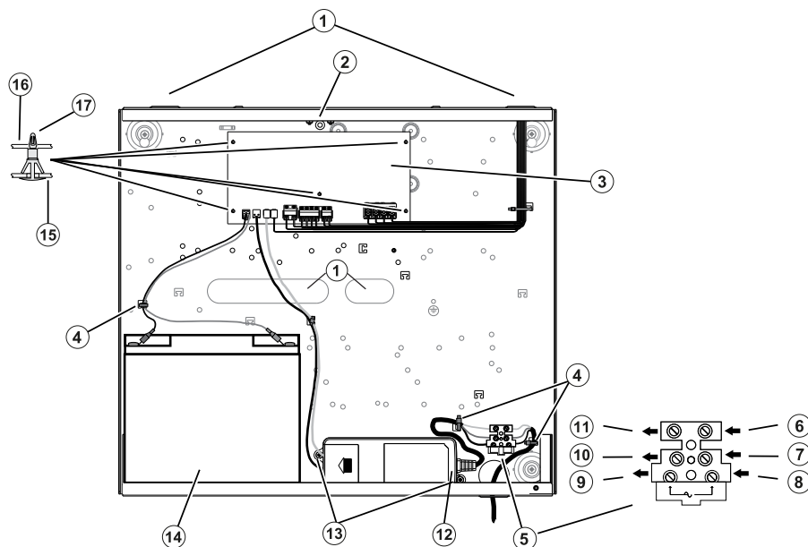
Abbildung 20: HSM3350-Verdrahtung für HSC3020C-Gehäuse
