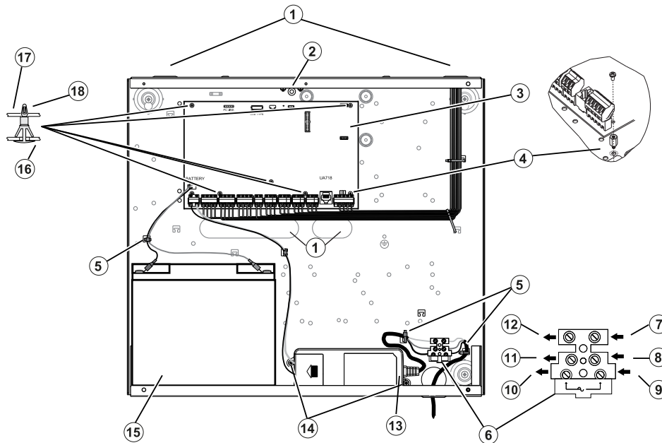
Abbildung 16: Schalttafelverdrahtung für HSC3020C (EU)-Gehäuse
