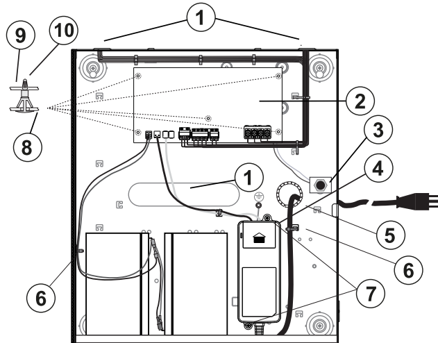
Abbildung 14: HSM3350 im Gehäuse HSC3010C
