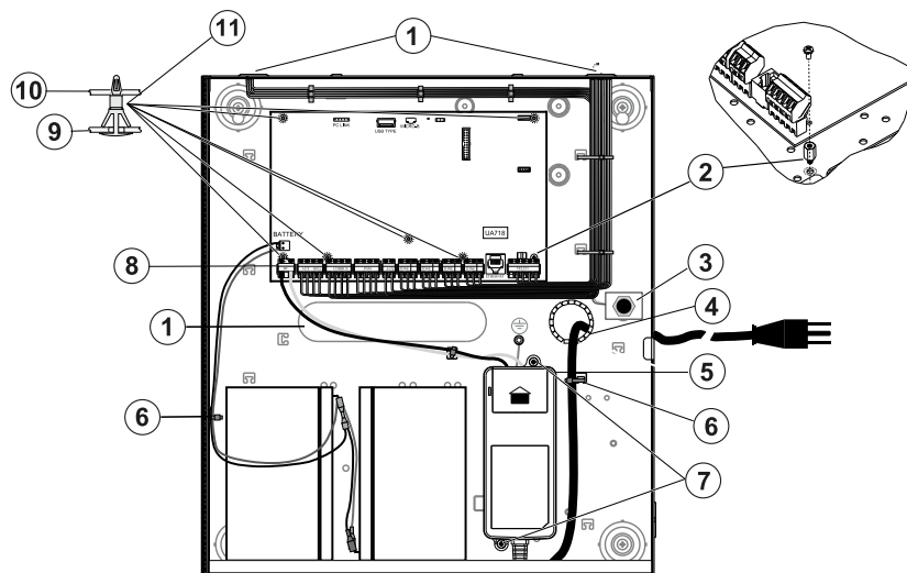
Abbildung 9: Verkabelung der Zentrale für HSC3010C
