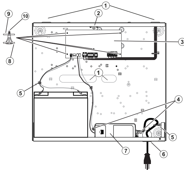
Abbildung 15: Nordamerikanisches Anschlussdiagramm für HSM3350 im HSC3020C-Gehäuse
