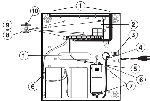
Abbildung 12: HSM3204CX im Gehäuse HSC3010C
