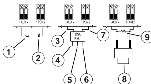
Abbildung 35: LED-Ausgang mit Strombegrenzungswiderstand und optionalem Relais-treiber-ausgang.
