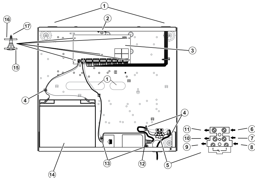
Abbildung 19: HSM3204CX-Verdrahtung für HSC3020C-Gehäuse
