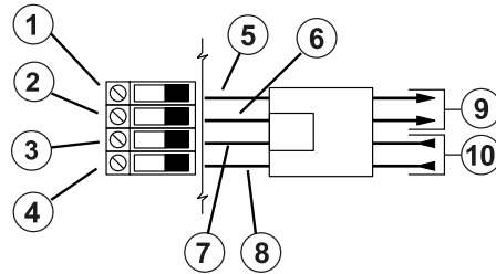
Abbildung 37: Telefonleitung-Anschluss
