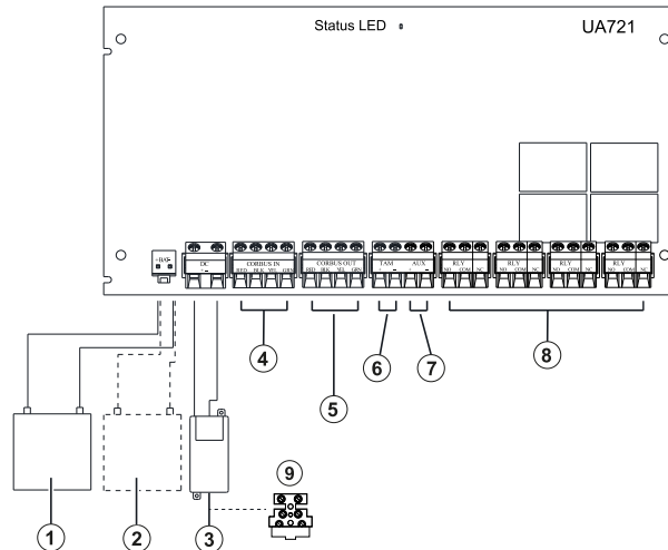
Abbildung 29: HSM3204CX Corbus Repeater
