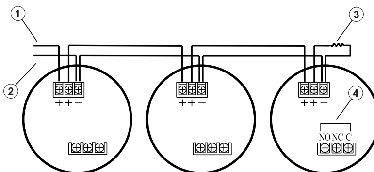
Abbildung 39: Verdrahtung 2-Draht-Rauchmelder
