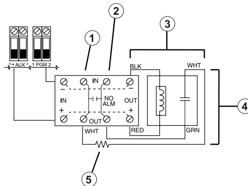
Abbildung 40: Verkabelung 4-Draht-Rauchmelder
