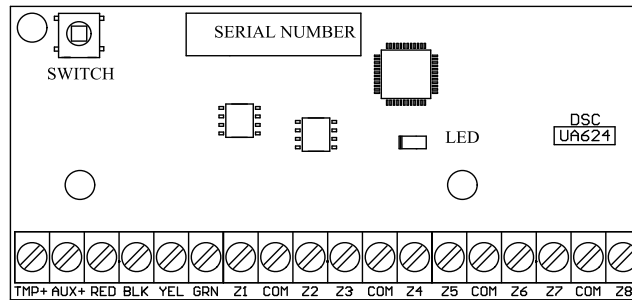
Abbildung 23: HSM3408 8-Linienerweiterung
