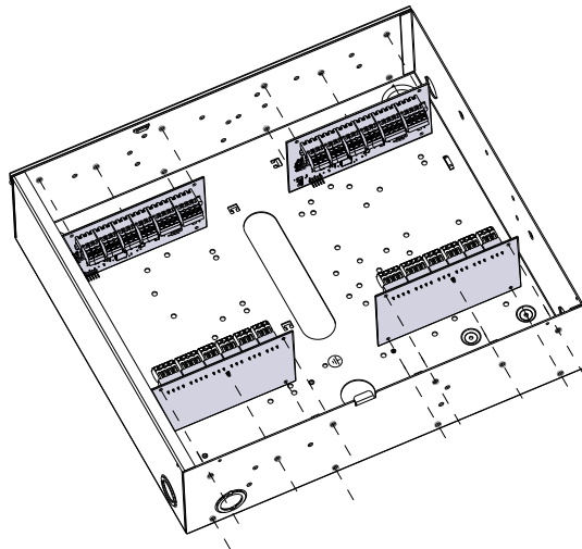
Abbildung 6: HSM3408 im Gehäuse HSC3010C
