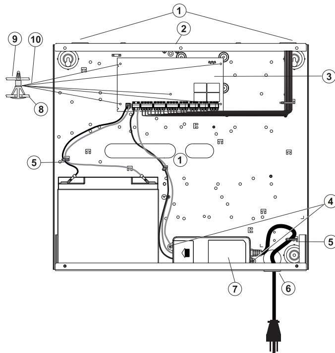
Abbildung 13: Nordamerikanisches Anschlussdiagramm für HSM3204CX im HSC3020C-Gehäuse
