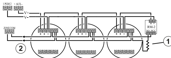
Abbildung 38: Rauchmelderverkabelung
