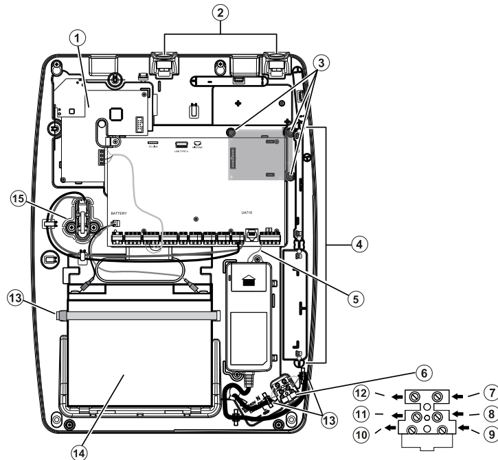
Abbildung 18: HSC3020CP Verkabelung
