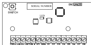
Abbildung 25: HSM2208 Ausgang Erweiterung
