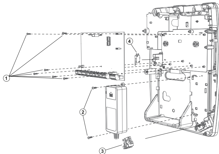
Abbildung 17: Installieren von Komponenten im HSC3020CP-Gehäuse
