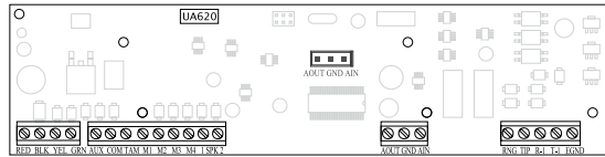
Abbildung 24: HSM2955 2-Wege-Audiomodul
